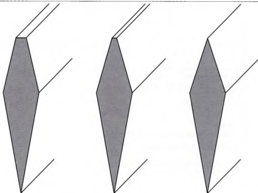
Поперечные сечения клинков сабли дао эпохи династии Мин без обозначенных линий ковки различных сортов железа. В Японии первые два типа сечения называются унокуби-цукури (unokubi-zukuri), а третий — моро-ха (moro-ha).
